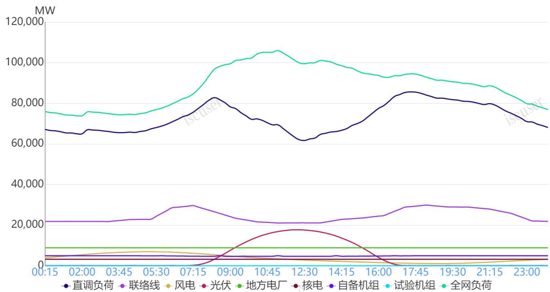
图 1 1 月 5 日负荷及电源出力预测情况
