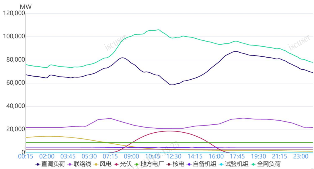
图 1 1月7日负荷及电源出力预测情况
