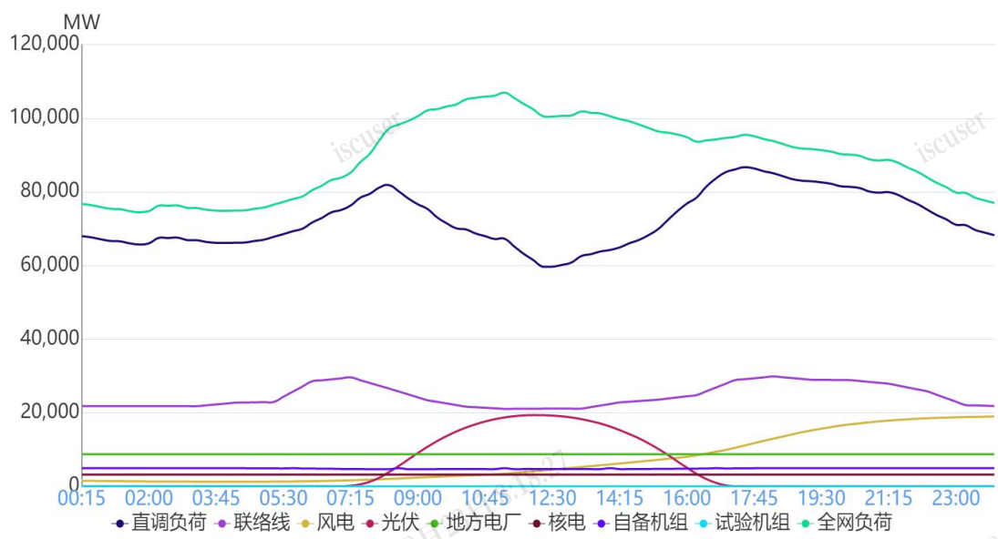
图 1 1月8日负荷及电源出力预测情况
