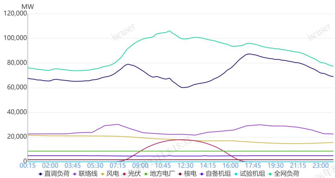
图 1 1月10日负荷及电源出力预测情况
