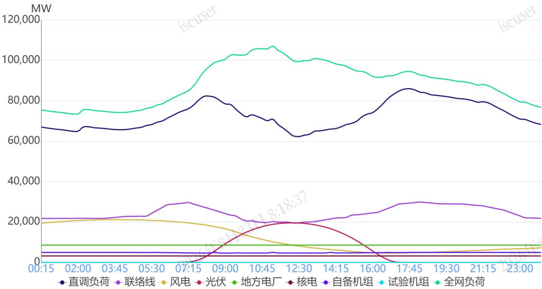
图 1 1月12日负荷及电源出力预测情况
