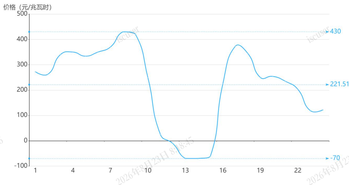
图2 1月15日日前市场用电侧价格
