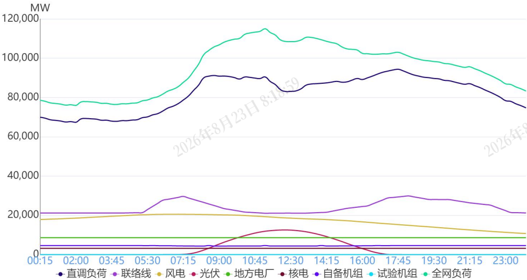
图 1 1月19日负荷及电源出力预测情况
