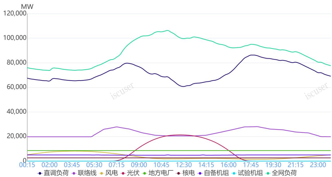
图 1 2 月 2 日负荷及电源出力预测情况
