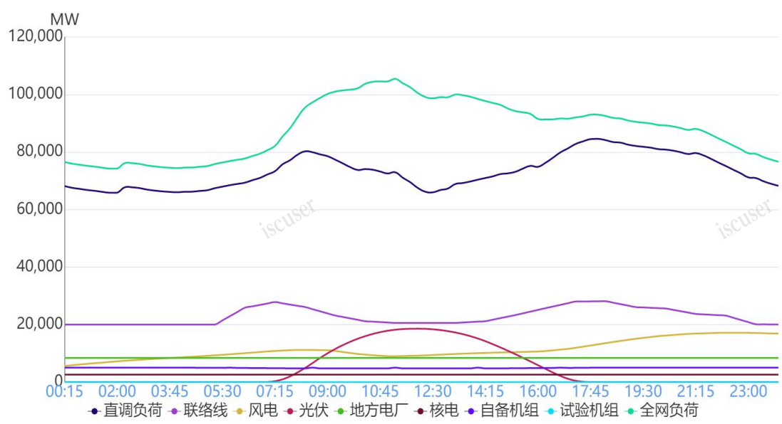
图 1 2 月 3 日负荷及电源出力预测情况
