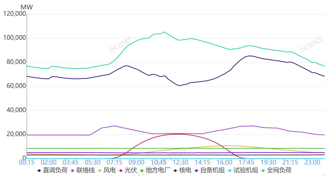
图 1 2月7日负荷及电源出力预测情况
