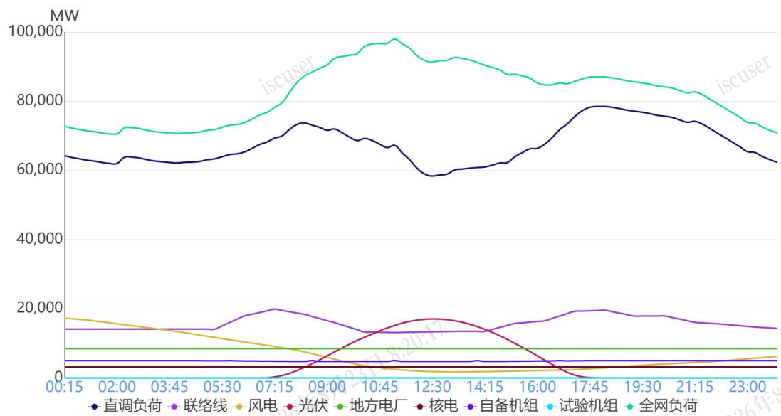
图 1 2月10日负荷及电源出力预测情况
