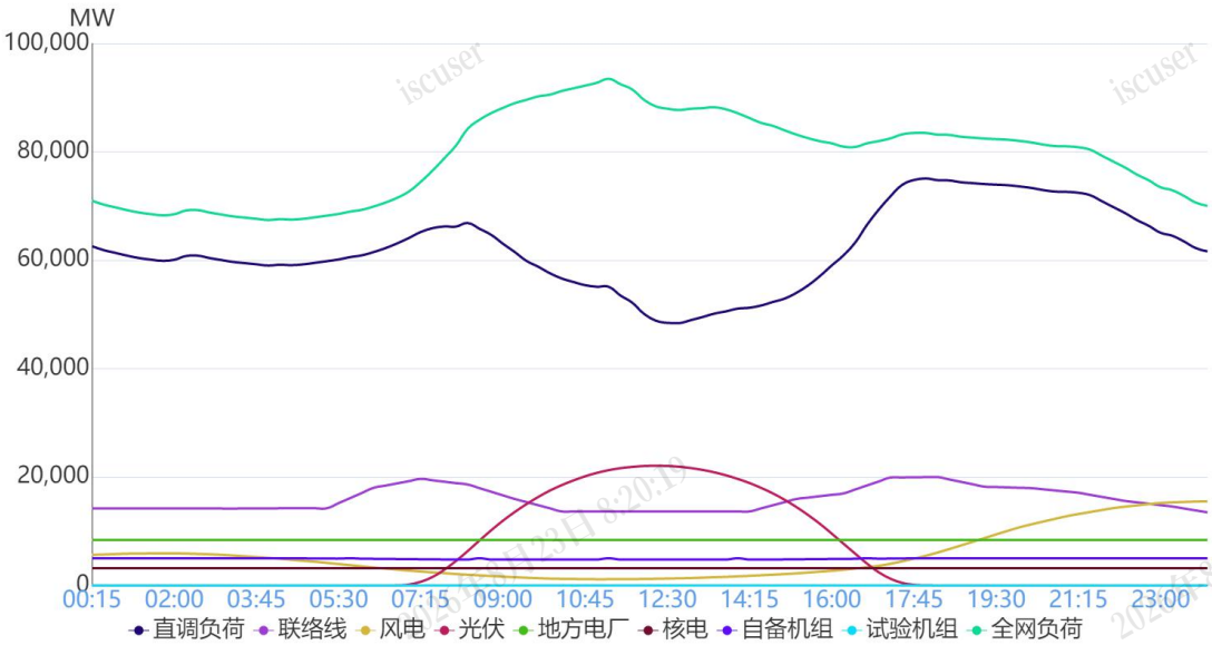
图 1 2月11日负荷及电源出力预测情况
