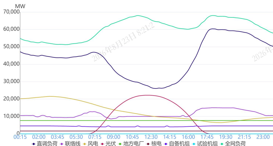
图 1 2月22日负荷及电源出力预测情况
