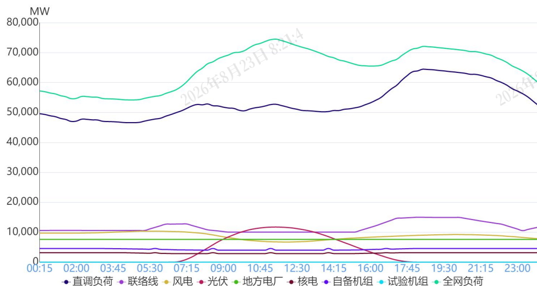
图 1 2月23日负荷及电源出力预测情况
