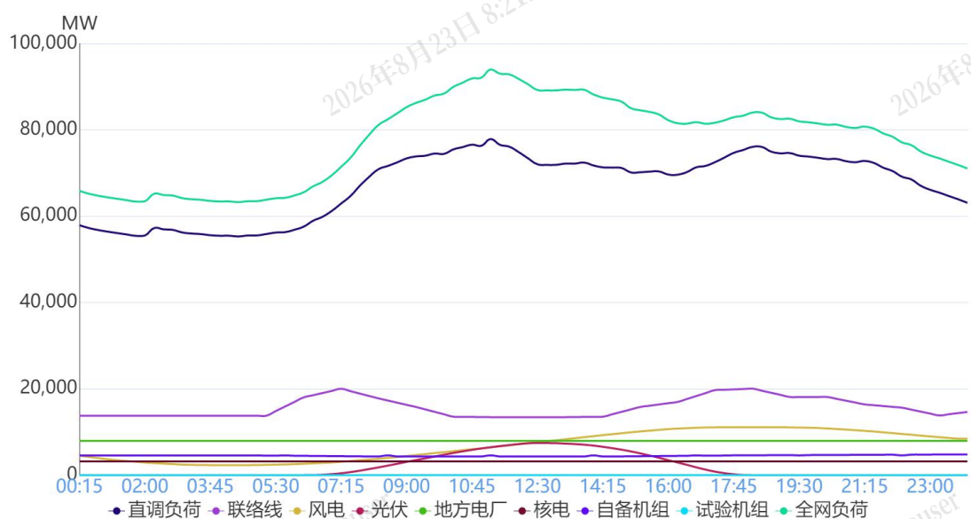
图 1 2月26日负荷及电源出力预测情况
