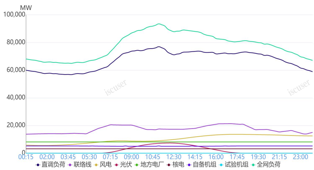
图 1 3 月 1 日负荷及电源出力预测情况
