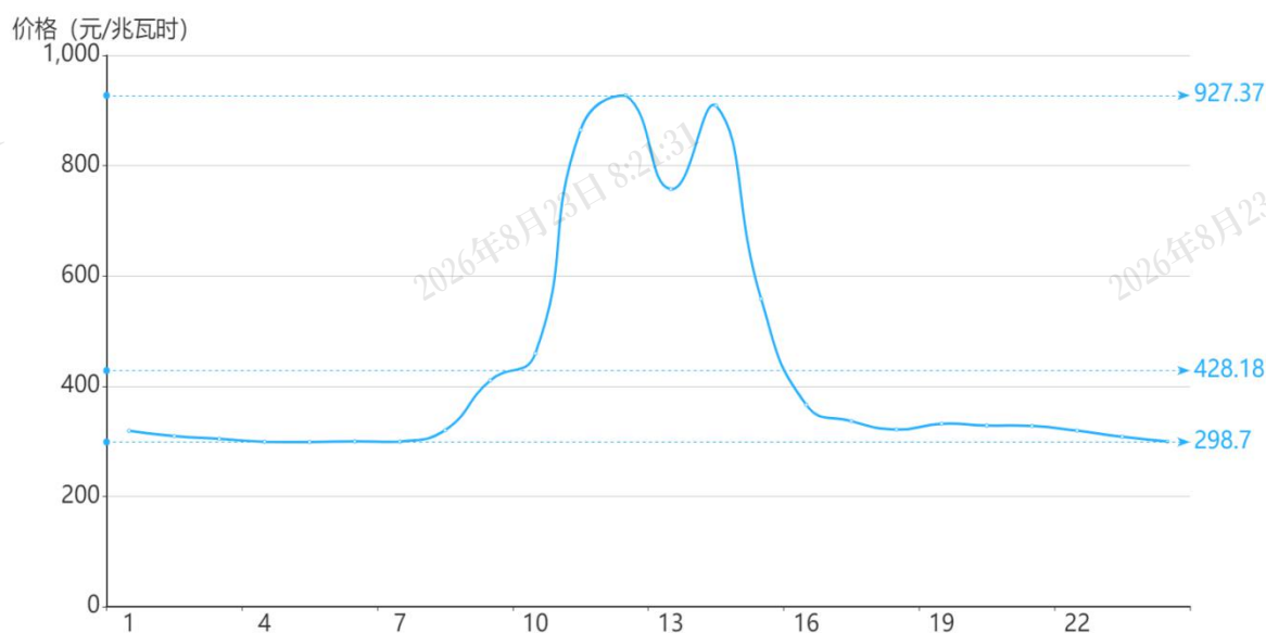
图 3 3 月 1 日实时市场用电侧价格
