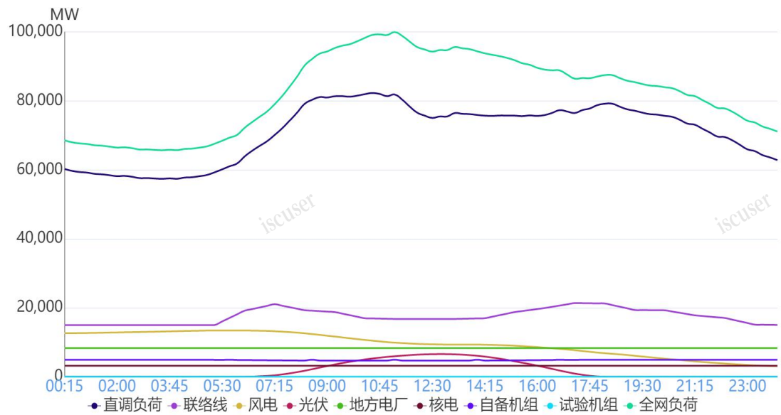
图 1 3 月 2 日负荷及电源出力预测情况
