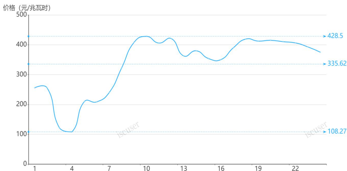
图2 3月2日日前市场用电侧价格
