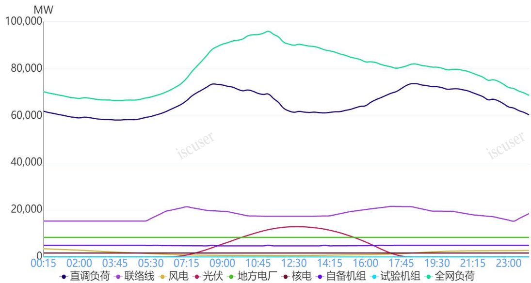
图 1 3 月 3 日负荷及电源出力预测情况
