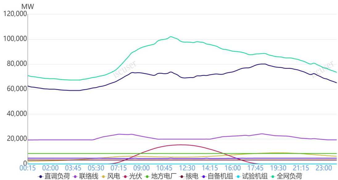
图 1 3 月 4 日负荷及电源出力预测情况
