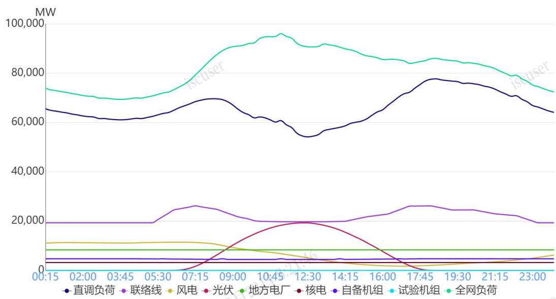
图 1 3月8日负荷及电源出力预测情况
