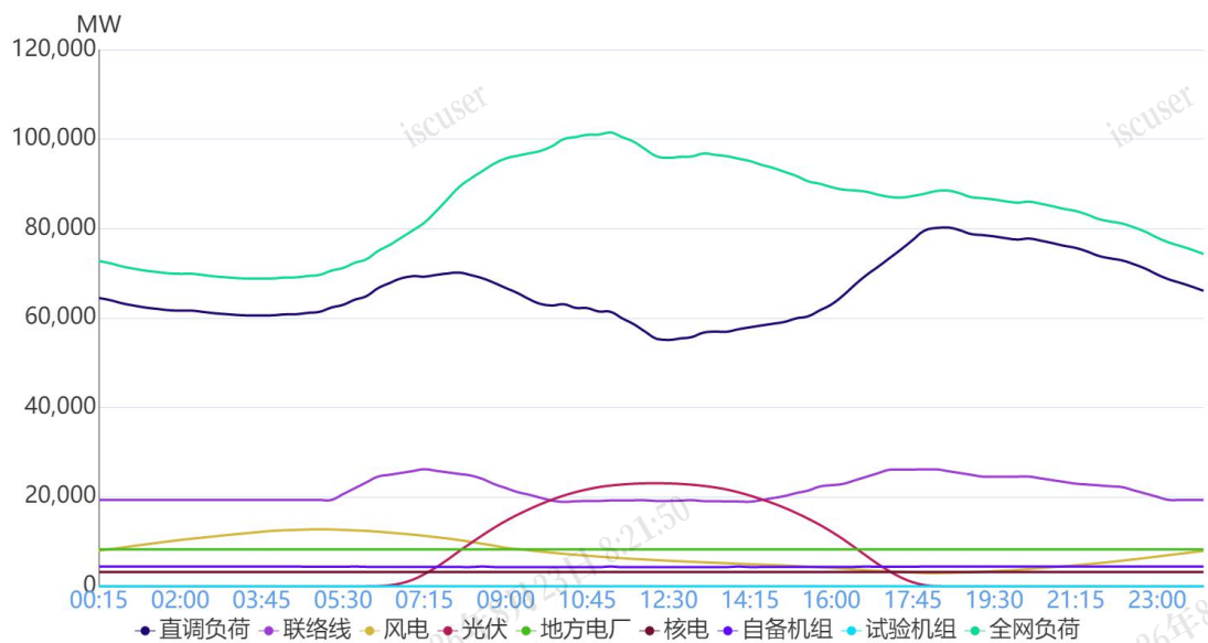
图 1 3月9日负荷及电源出力预测情况
