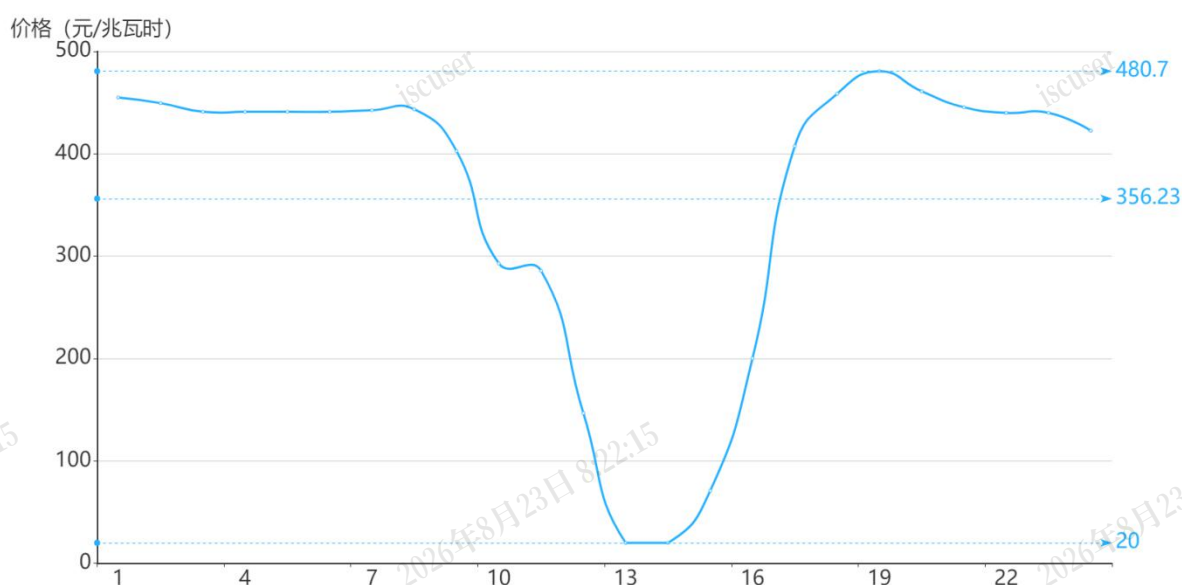
图2 3月16日日前市场用电侧价格
