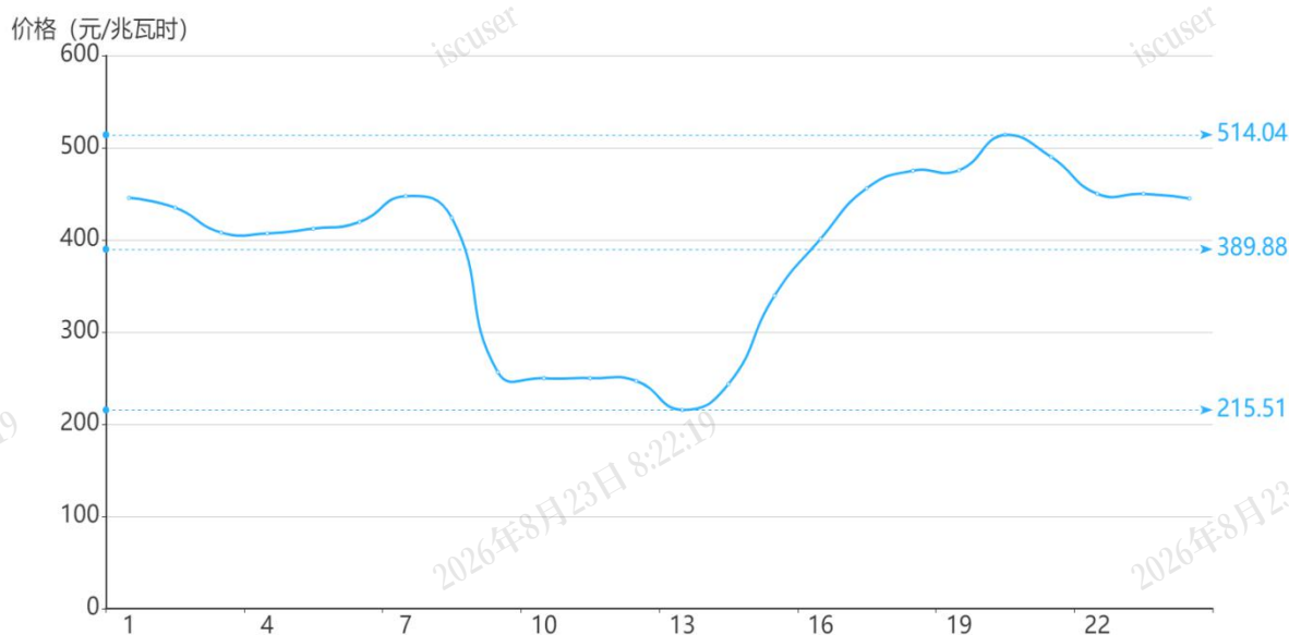
图2 3月17日日前市场用电侧价格
