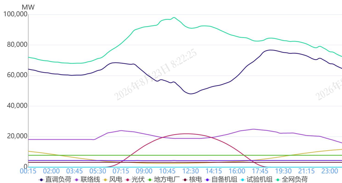
图 1 3月20日负荷及电源出力预测情况
