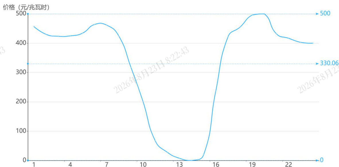
图 2 3 月 24 日日前市场用电侧价格
