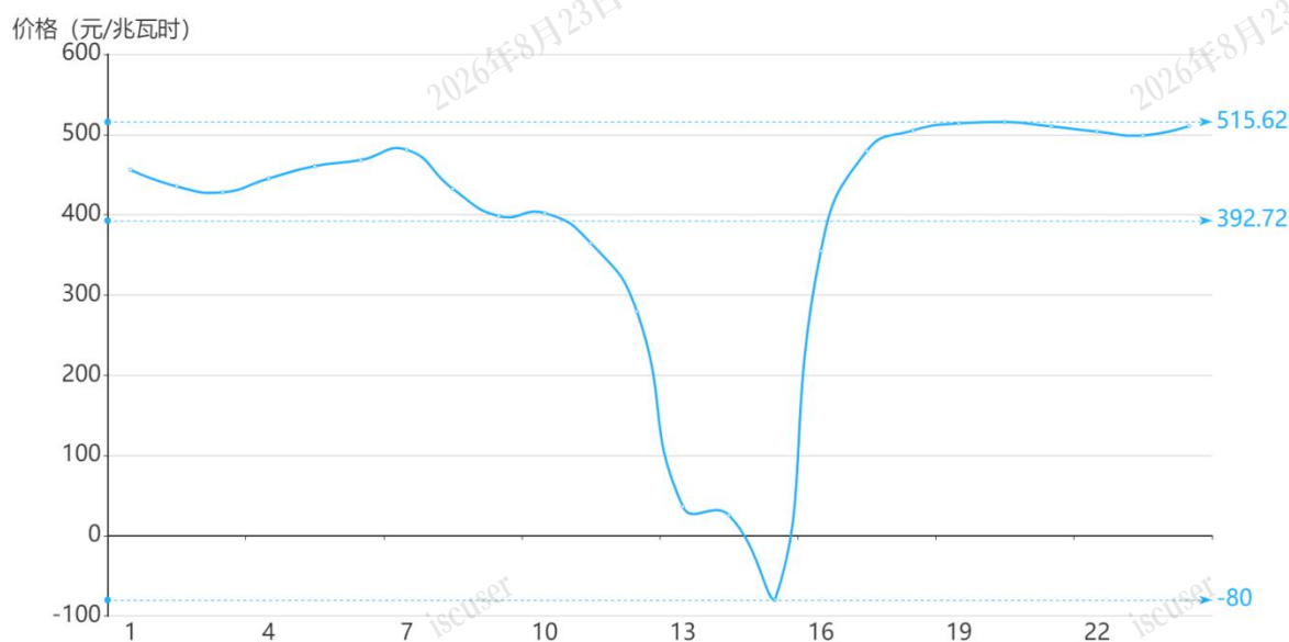
图 3 3 月 23 日实时市场用电侧价格
