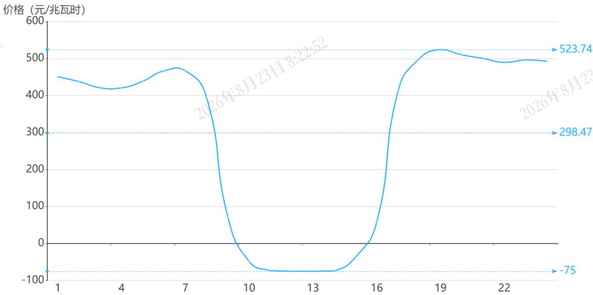
图 2 3 月 27 日日前市场用电侧价格
