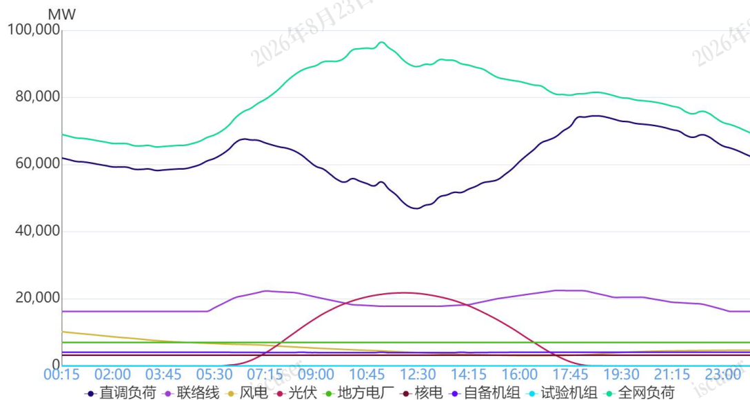
图1 3月27日负荷及电源出力预测情况
