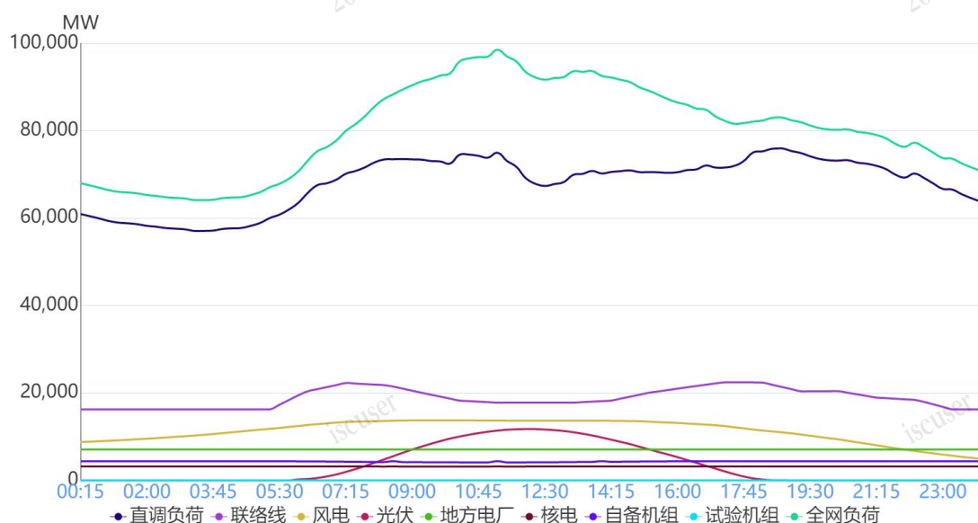
图1 3月30日负荷及电源出力预测情况
