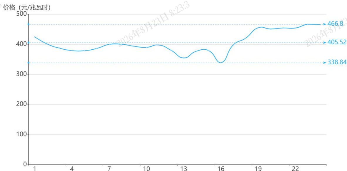
图 2 3 月 30 日日前市场用电侧价格
