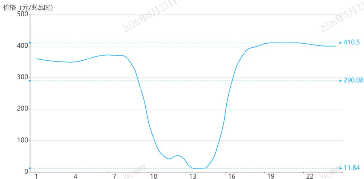
图 2 3 月 31 日日前市场用电侧价格
