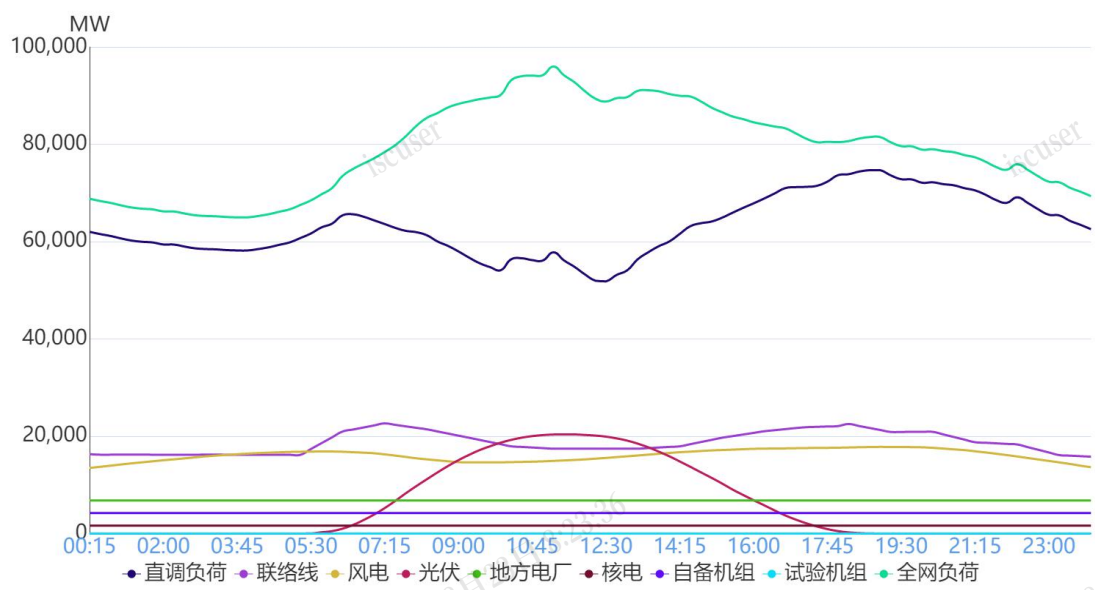
图 1 4月8日负荷及电源出力预测情况
