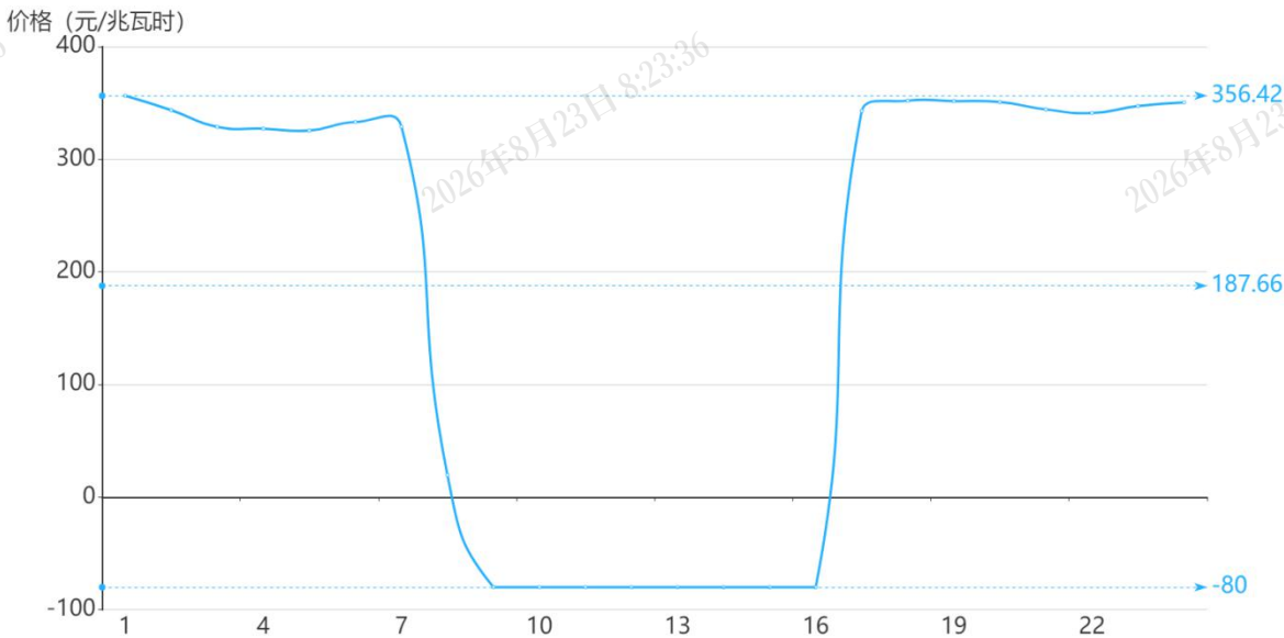
图 3 4 月 7 日实时市场用电侧价格
