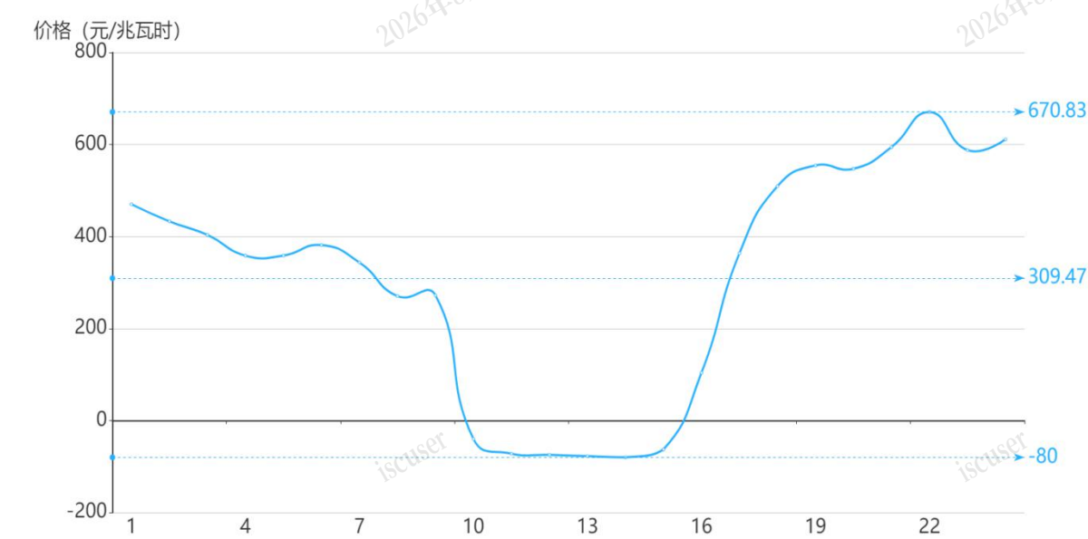
图 3 4 月 13 日实时市场用电侧价格
