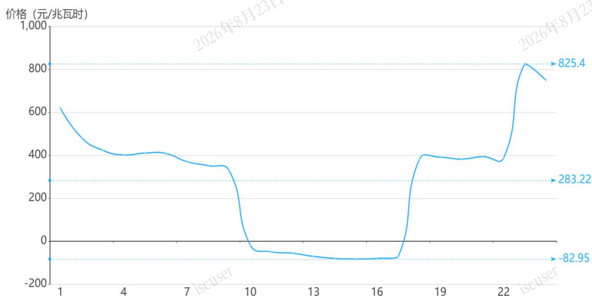
图3 4月27日实时市场用电侧价格
