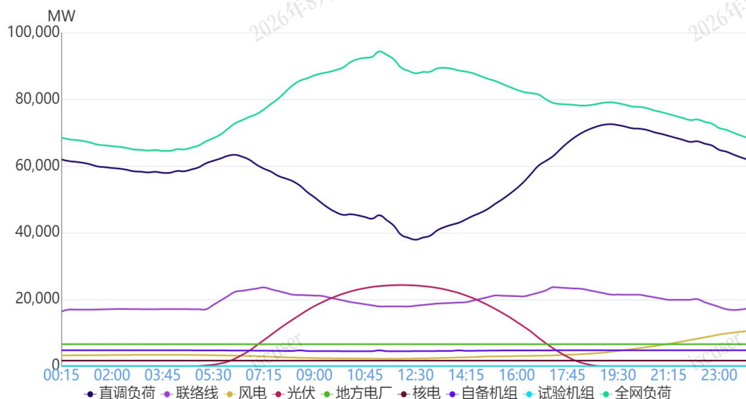
图 1 4月29日负荷及电源出力预测情况
