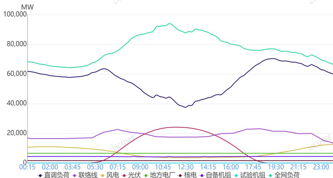
图 1 4月30日负荷及电源出力预测情况
