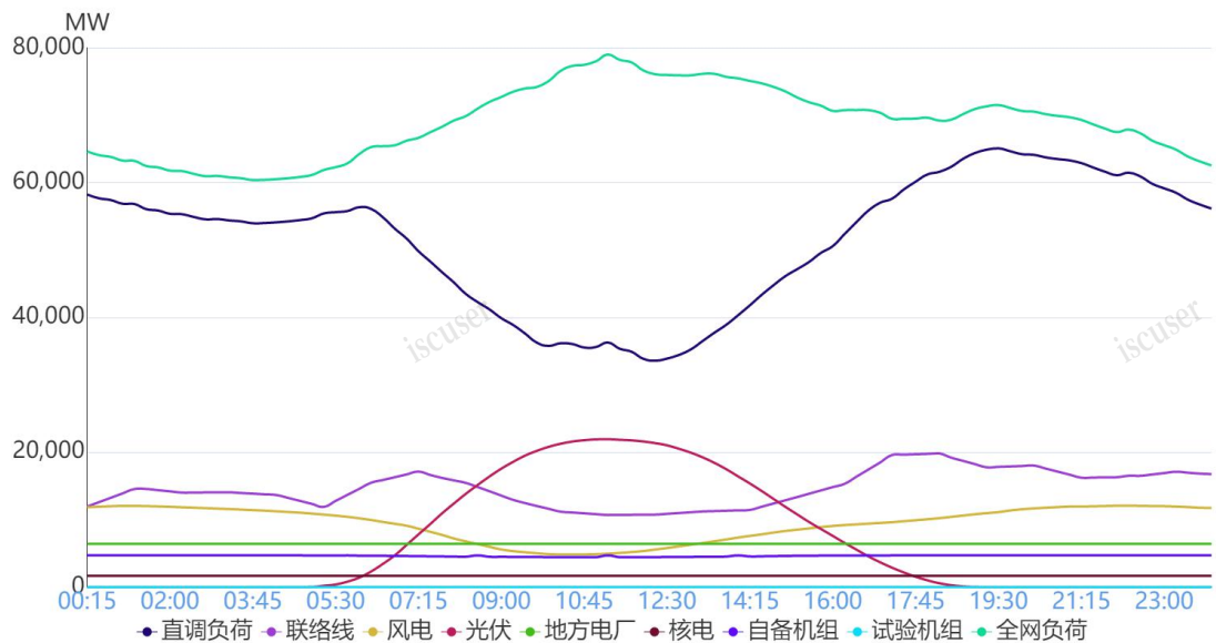
图 1 5 月 1 日负荷及电源出力预测情况
