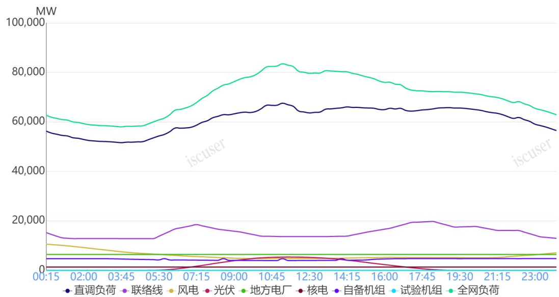
图 1 5 月 2 日负荷及电源出力预测情况
