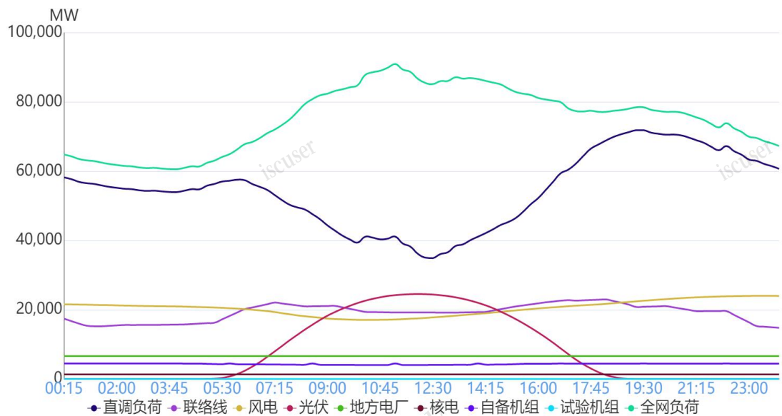
图 1 5 月 5 日负荷及电源出力预测情况
