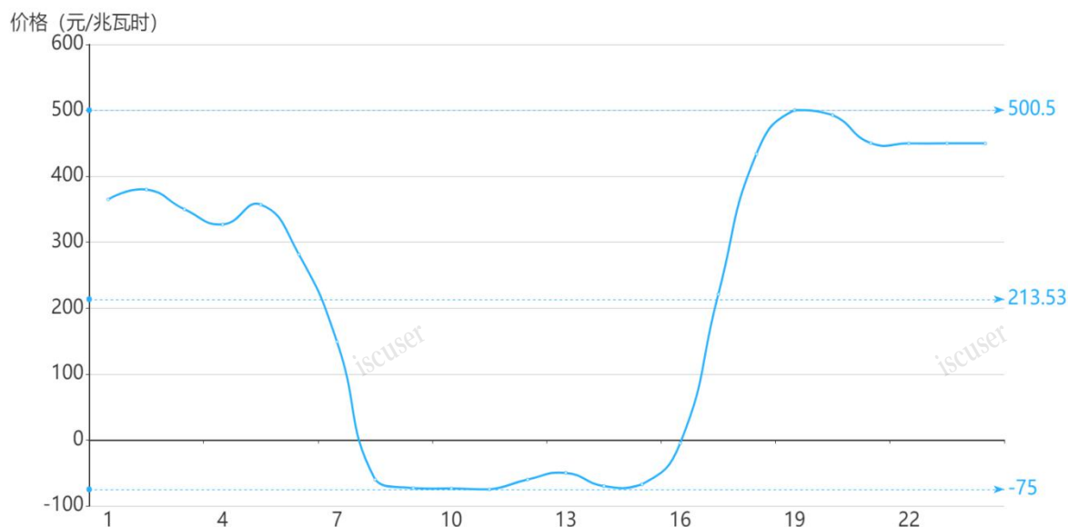
图2 5月5日日前市场用电侧价格
