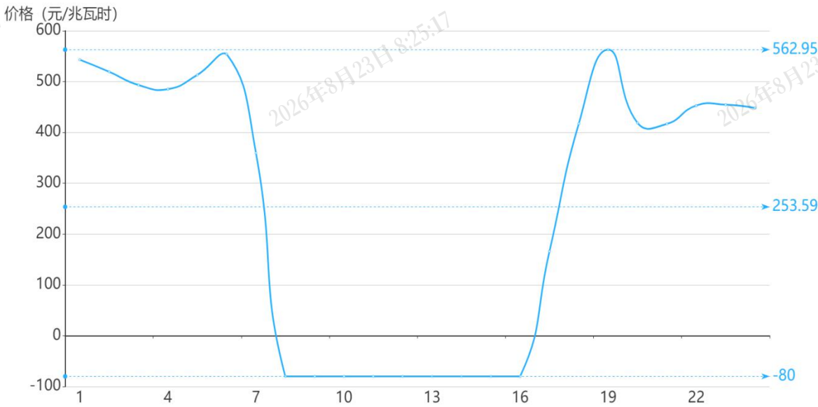
图 3 5 月 4 日实时市场用电侧价格
