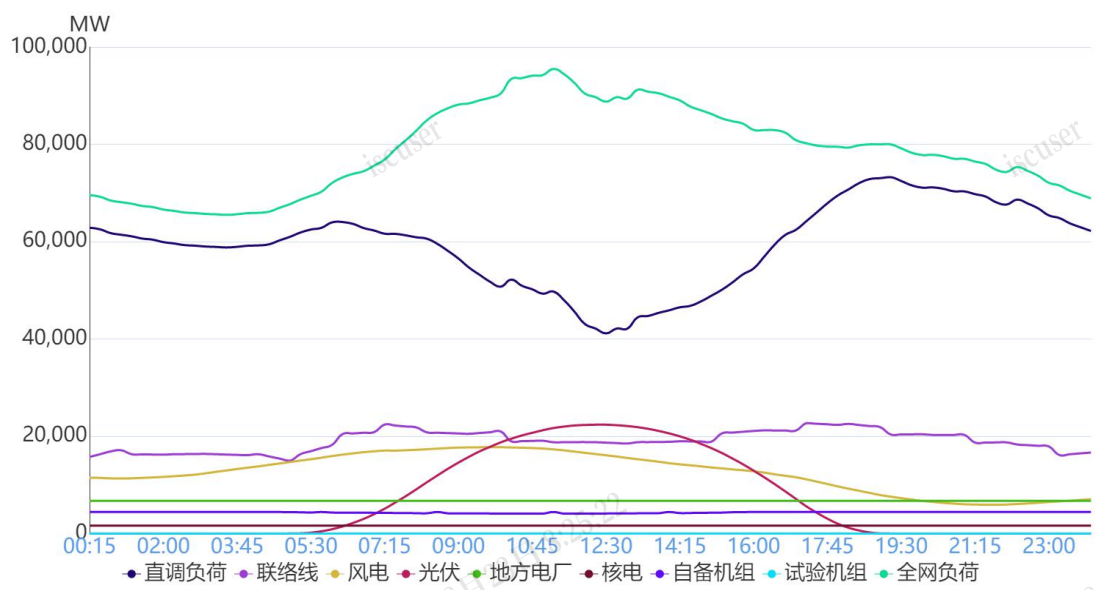
图 1 5月7日负荷及电源出力预测情况
