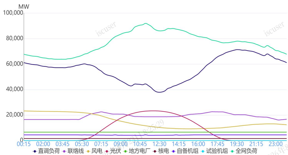
图 1 5月10日负荷及电源出力预测情况
