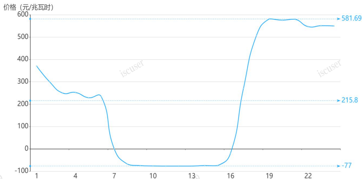
图2 5月10日日前市场用电侧价格
