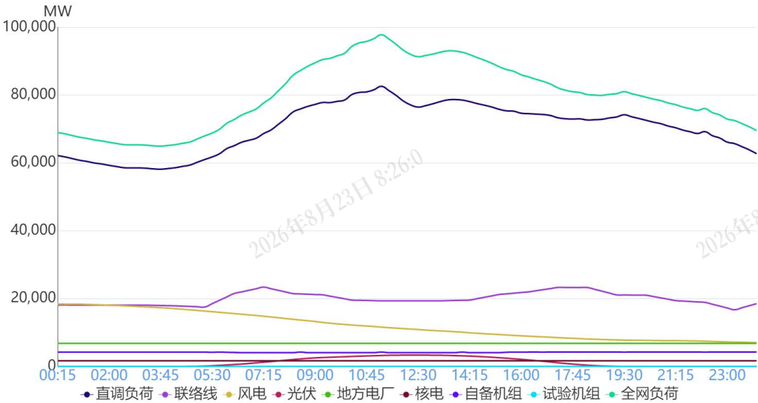
图1 5月18日负荷及电源出力预测情况
