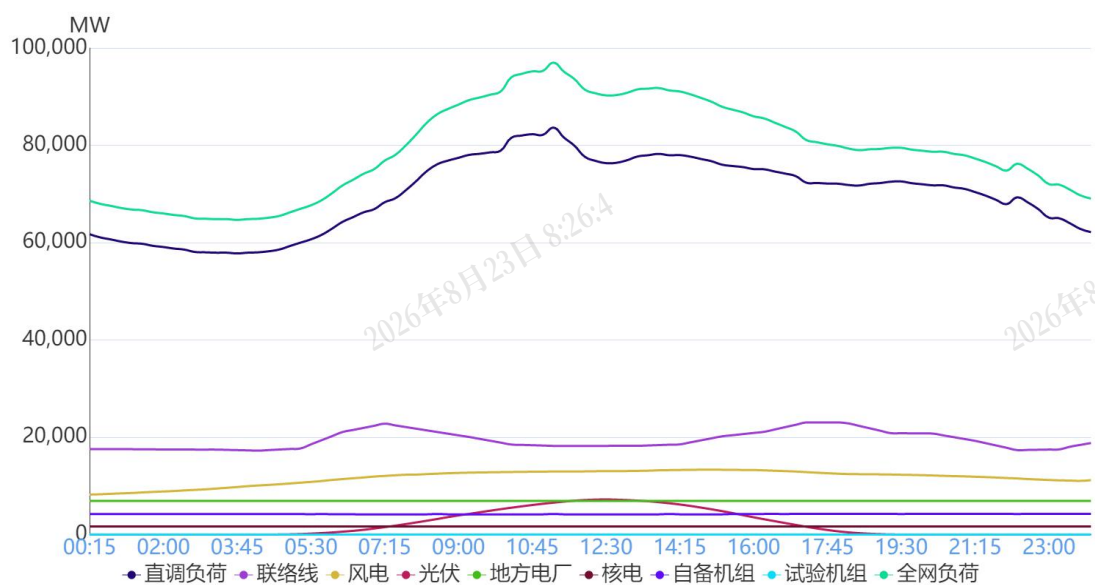
图 1 5月19日负荷及电源出力预测情况
