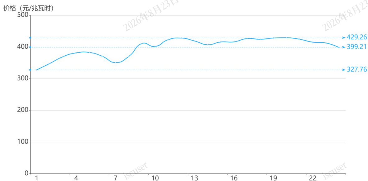
图3 5月18日实时市场用电侧价格
