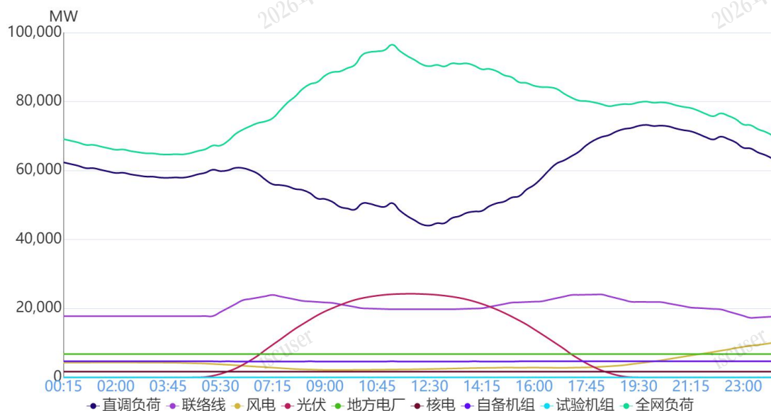
图 1 5月29日负荷及电源出力预测情况
