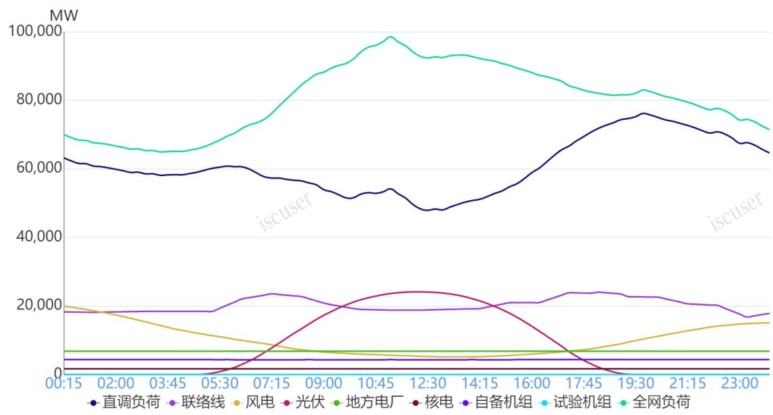
图 1 6 月 1 日负荷及电源出力预测情况
