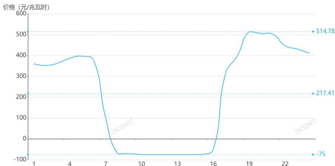
图2 6月1日日前市场用电侧价格
