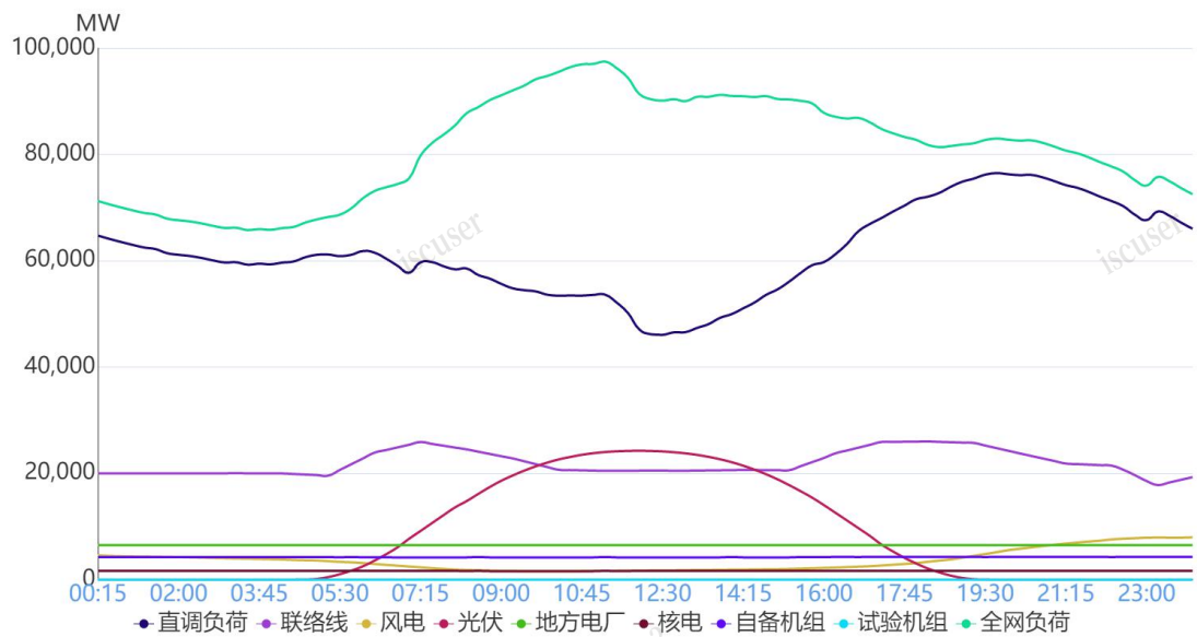
图 1 6 月 5 日负荷及电源出力预测情况
