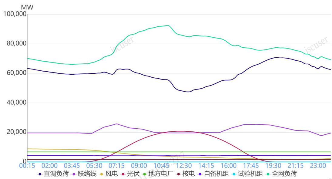
图 1 6月7日负荷及电源出力预测情况
