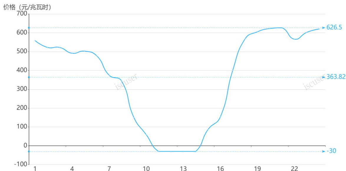
图2 6月7日日前市场用电侧价格
