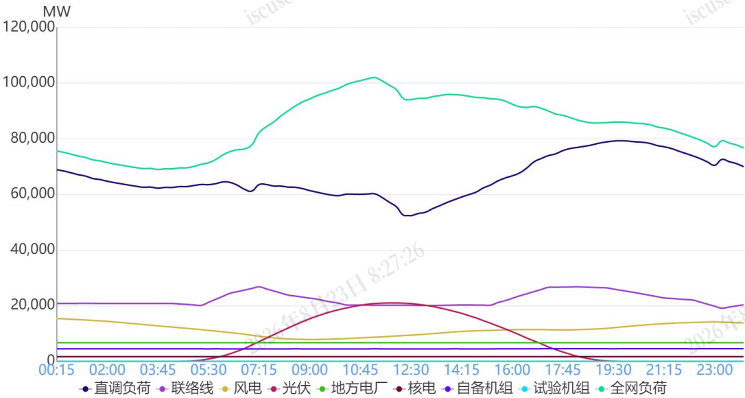
图 1 6月13日负荷及电源出力预测情况
