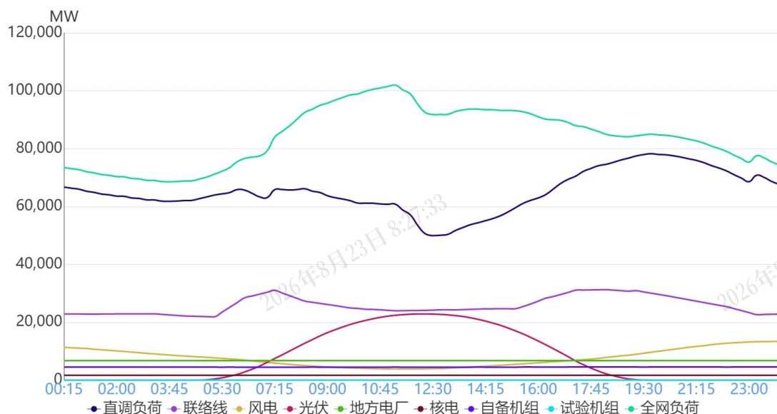
图1 6月16日负荷及电源出力预测情况
