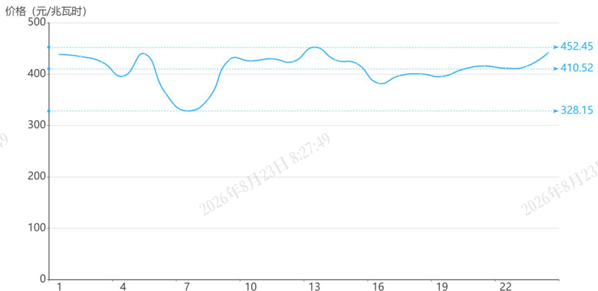
图2 6月21日日前市场用电侧价格
