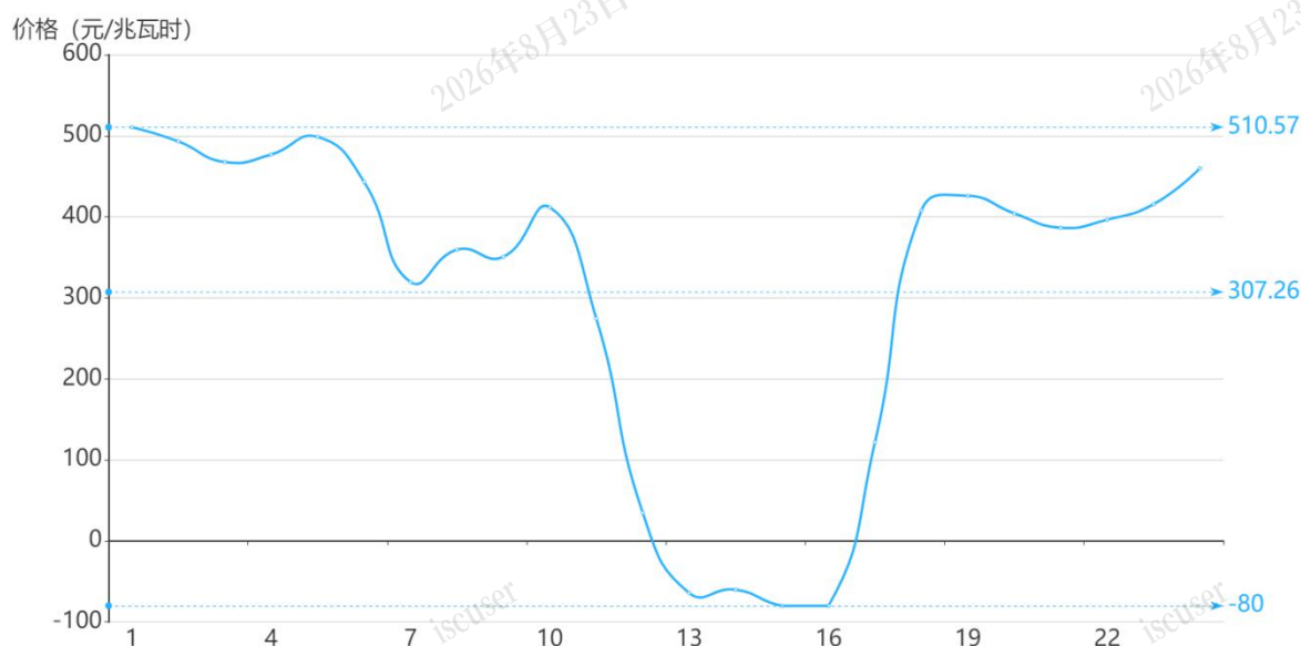
图3 6月22日实时市场用电侧价格
