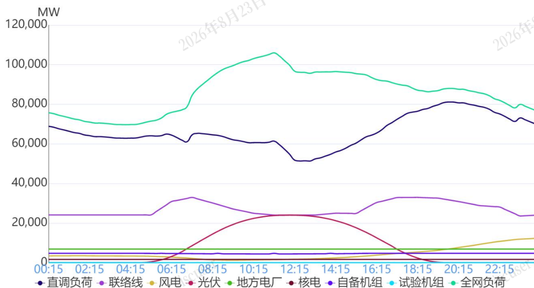
图 1 6月27日负荷及电源出力预测情况
