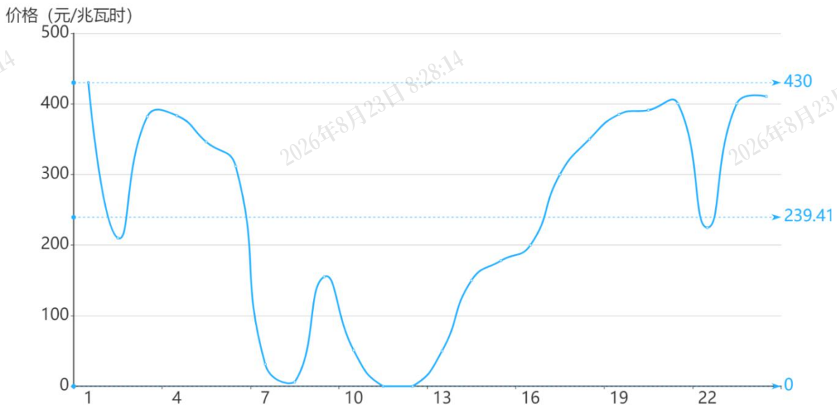
图 2 6 月 28 日日前市场用电侧价格
